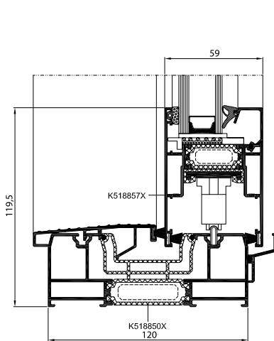
Doorsnede deur met een kozijn met 2 rails
