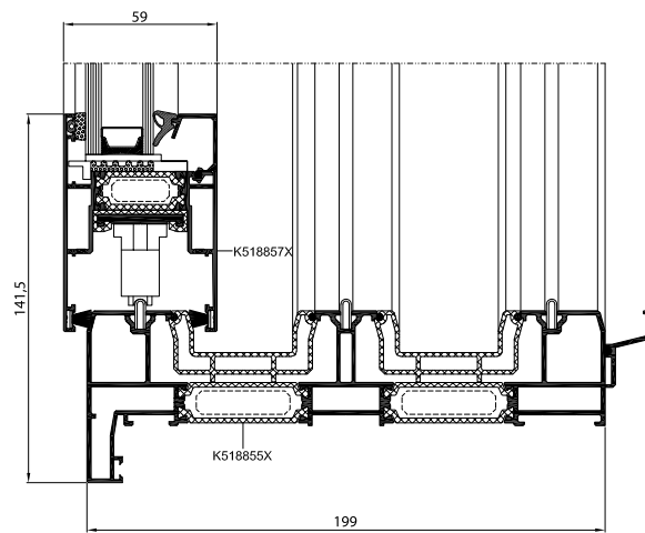
Doorsnede deur met een kozijn met 3 rails
