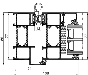
Sezione laterale della porta-finestra
